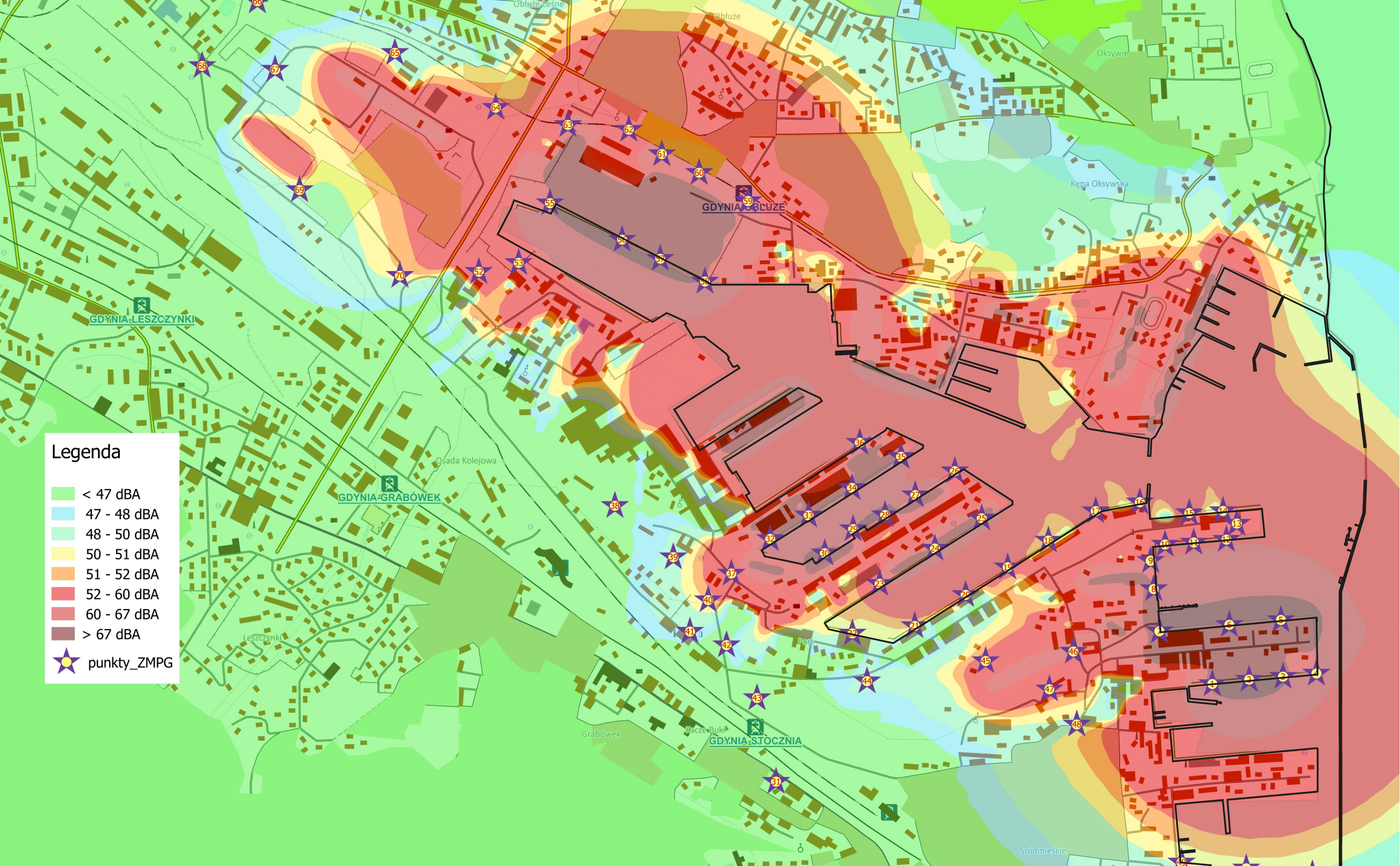
Okresowe pomiary poziomu hałasu w środowisku powodowanego pracą portu morskiego w Gdyni Załącznik 4.3 PORA DNIA
